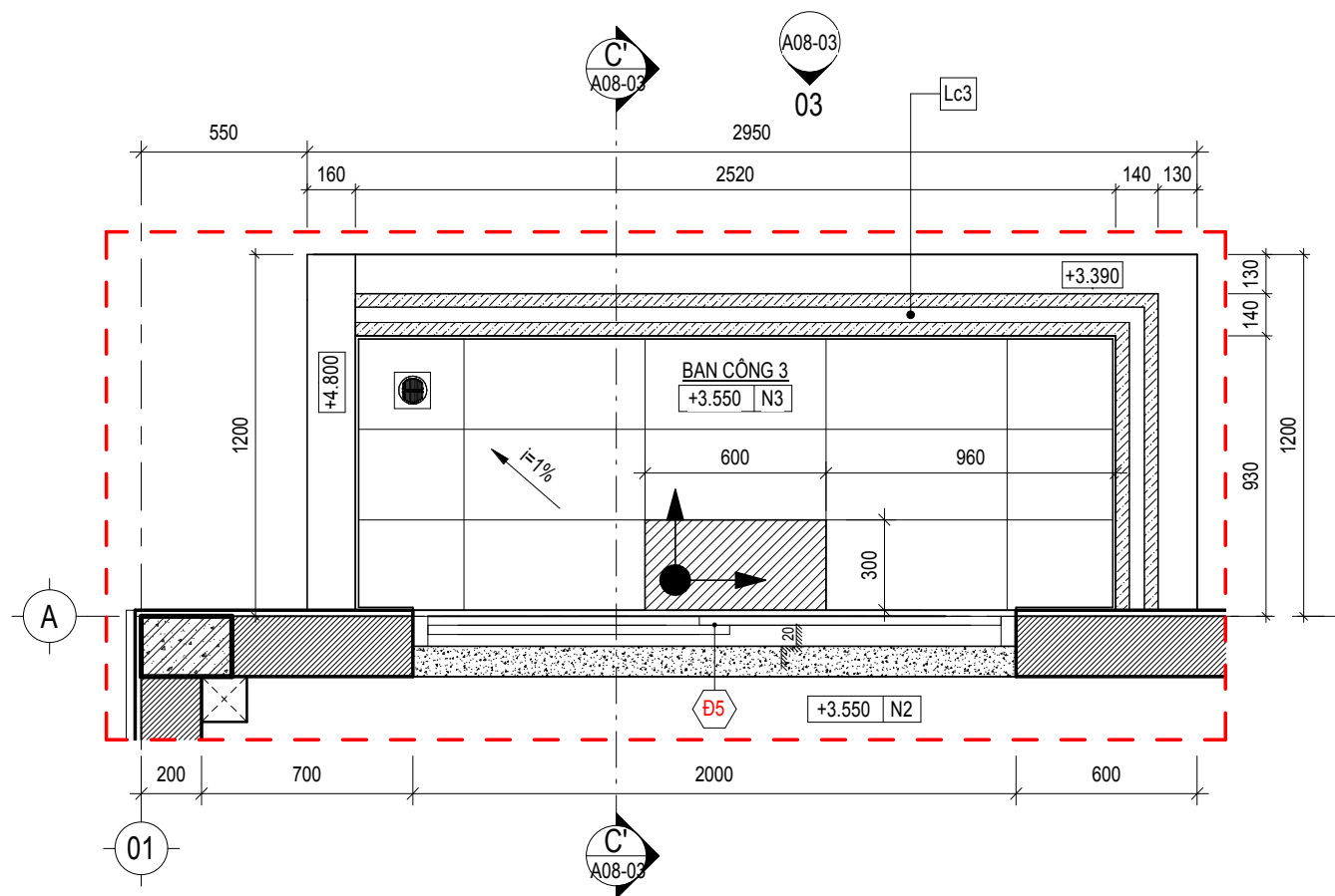
BC3 CT BAN CÔNG 3 (ĐIỂN HÌNH) - MẶT BẰNG TỶ LỆ 1 : 25
