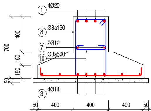
MC 1-1 PA1 - M2 (TL: 1/25)
