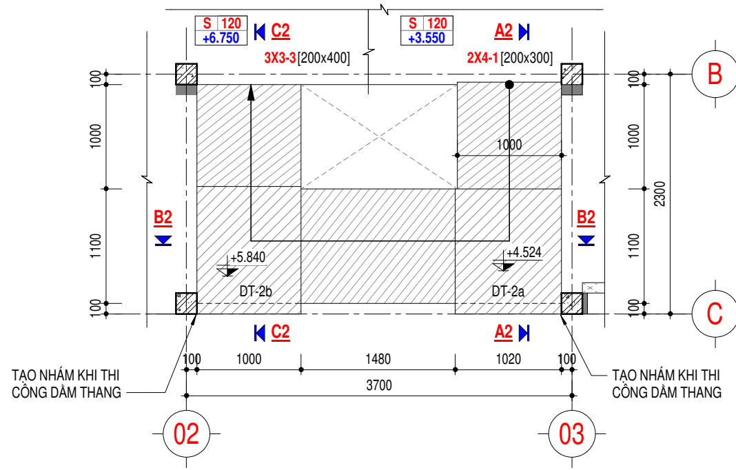
MẶT BẰNG CẦU THANG TẦNG 2 - TẦNG 3
