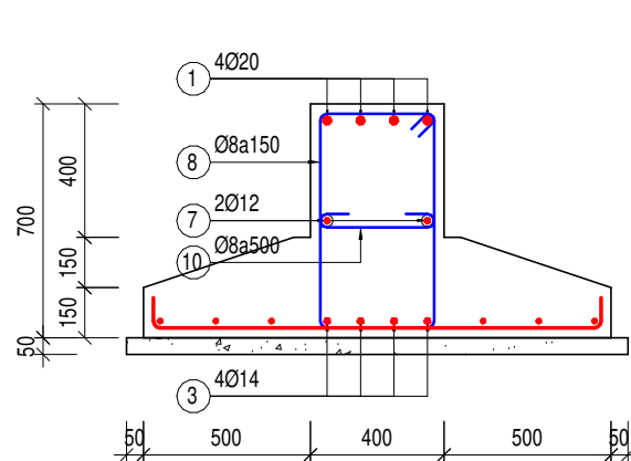
MC 1-1 PA2 - M2 (TL: 1/25)
