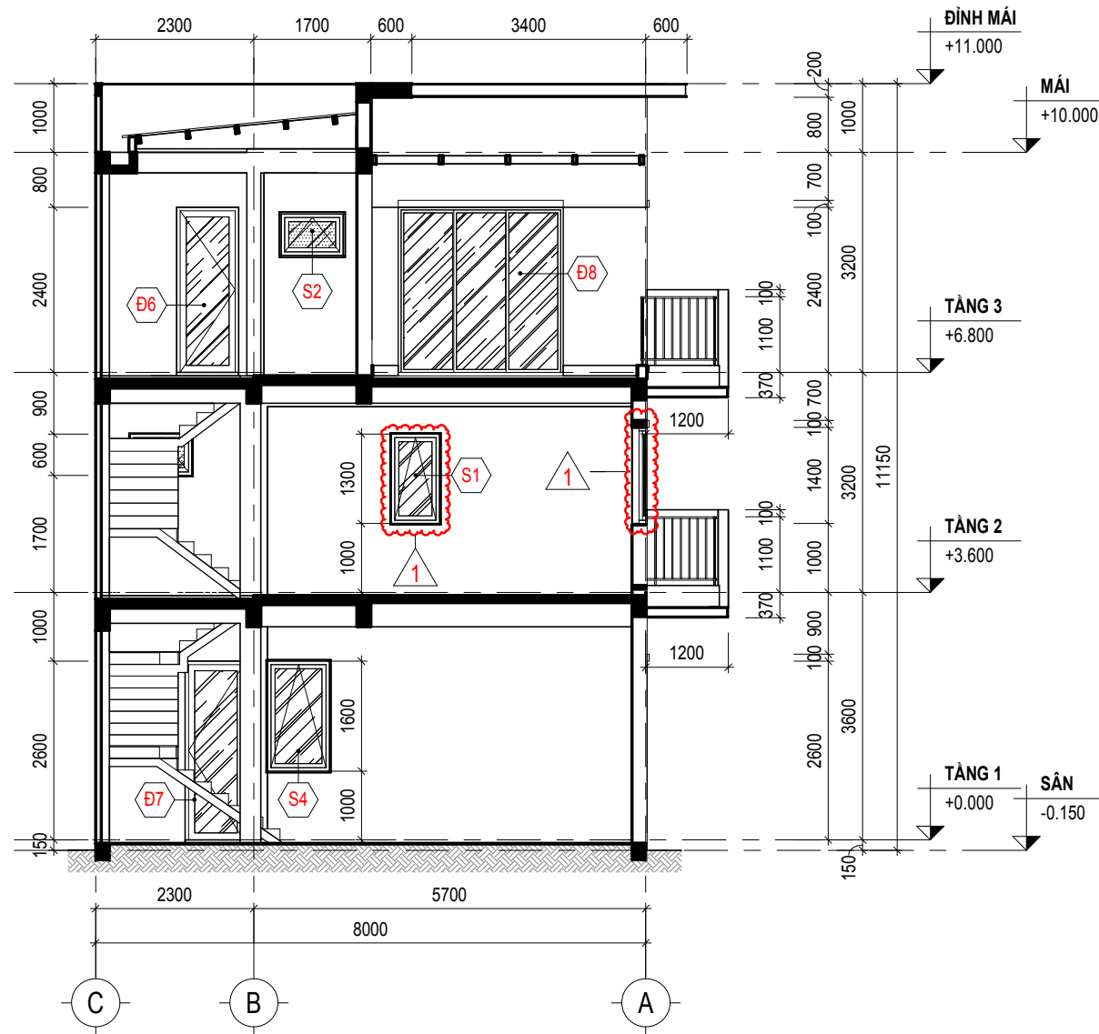
MẶT CẮT 2-2 TỶ LỆ 1:100
