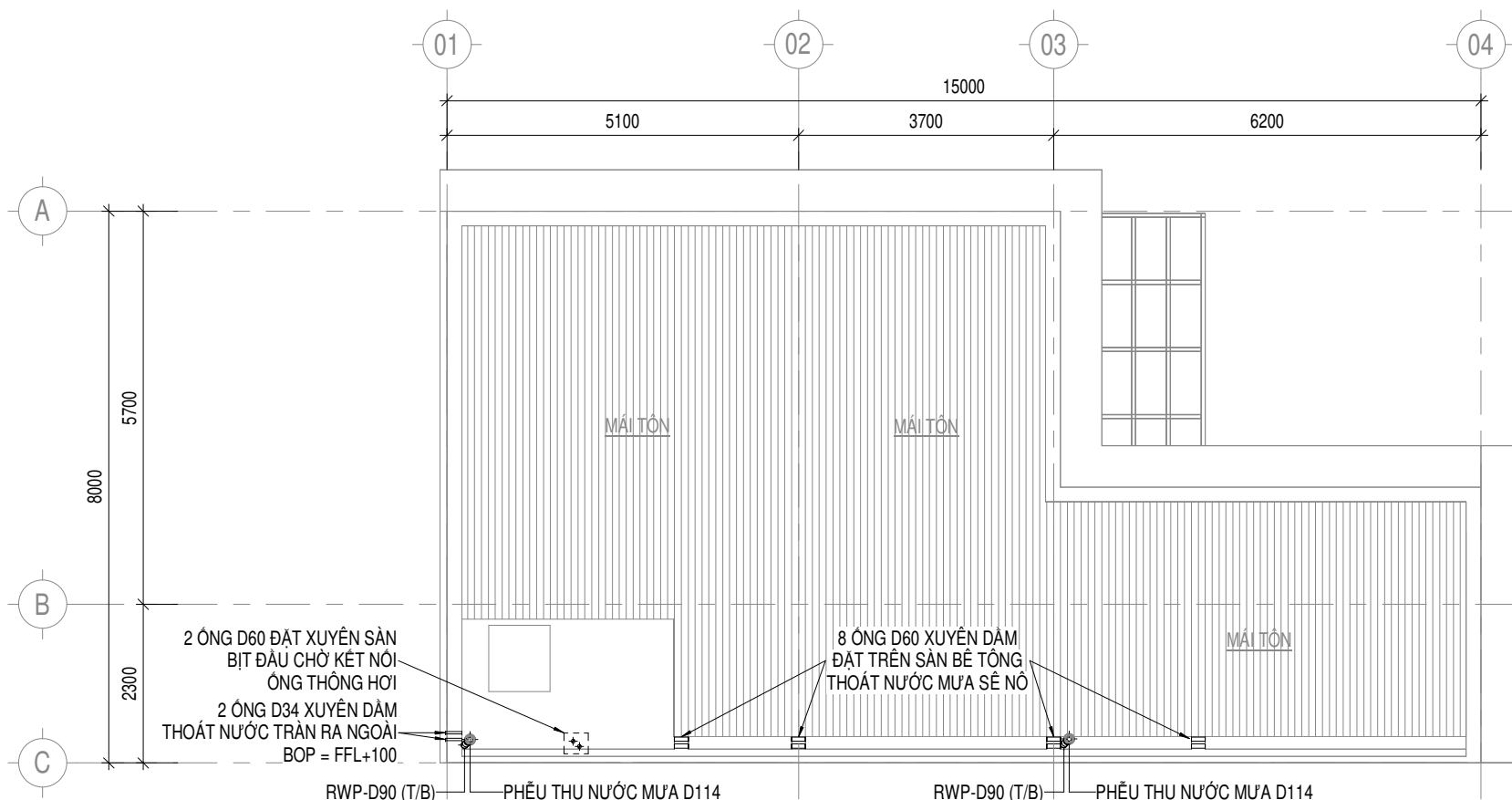
MẶT BẰNG CẤP THOÁT NƯỚC TẦNG MÁI TỶ LỆ 1 : 100
