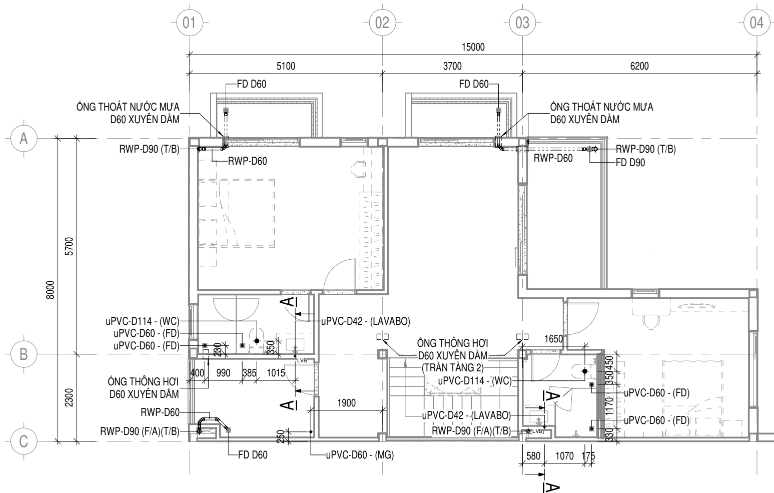
MẶT BẰNG CẤP THOÁT NƯỚC TẦNG 3 TỶ LỆ 1 : 100
