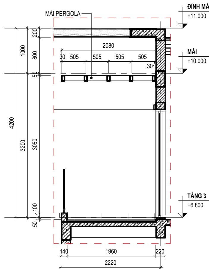
CHI TIẾT LAM MÁI - MẶT CẮT F' - 03 TỶ LỆ 1:50
