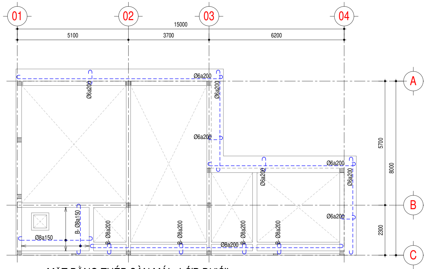
MẶT BẰNG THÉP SÀN MÁI - LỚP DƯỚI
