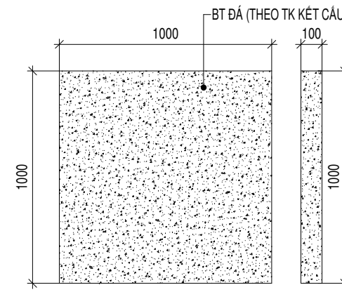
TẦM ĐẠN ĐÁY HỒ GA, TỶ LỆ 1/25 (TẦM ĐẠN 2)
