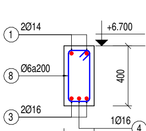
MC 4-4 3Y4 (TL: 1/25)
