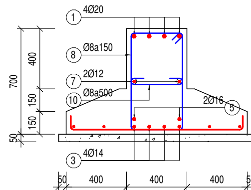
MC 3-3 PA1 - M2 (TL: 1/25)
