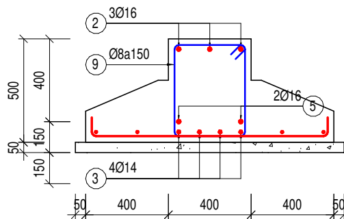
MC 4-4 PA1 - M2 (TL: 1/25)
