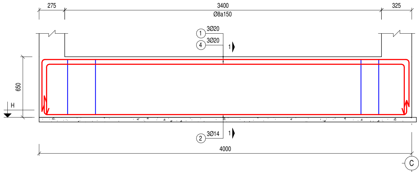
MÓNG PA2 - M4 (SL=1; L=4000)
