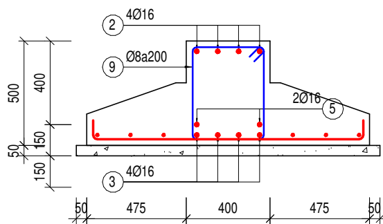
MC 4-4 PA1 - M3 (TL: 1/25)
