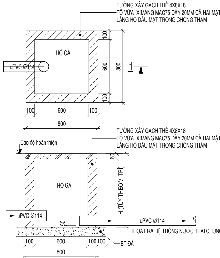
CHI TIẾT HỒ GA, TỶ LỆ 1/25
