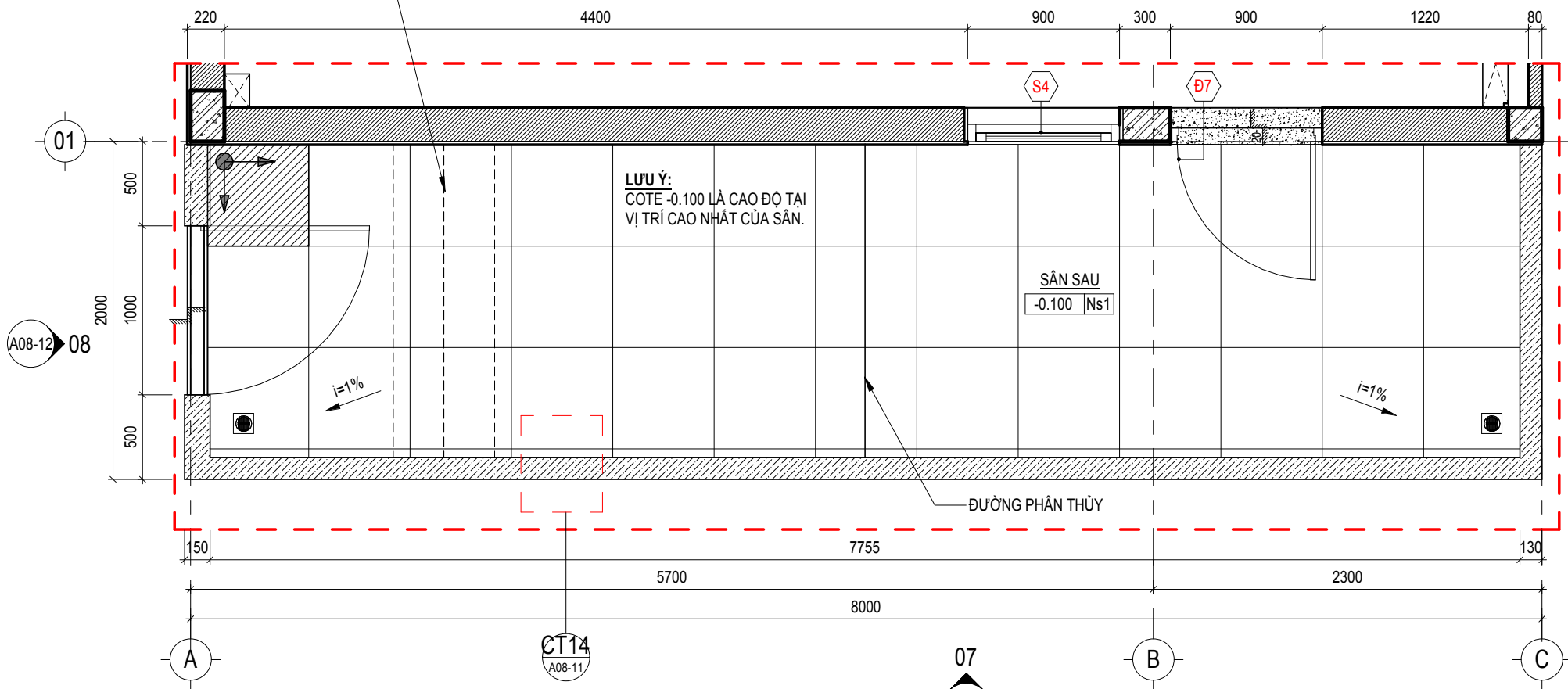
SS A02-51 CHI TIẾT SÂN SAU - MẶT BẰNG TỶ LỆ 1:35
