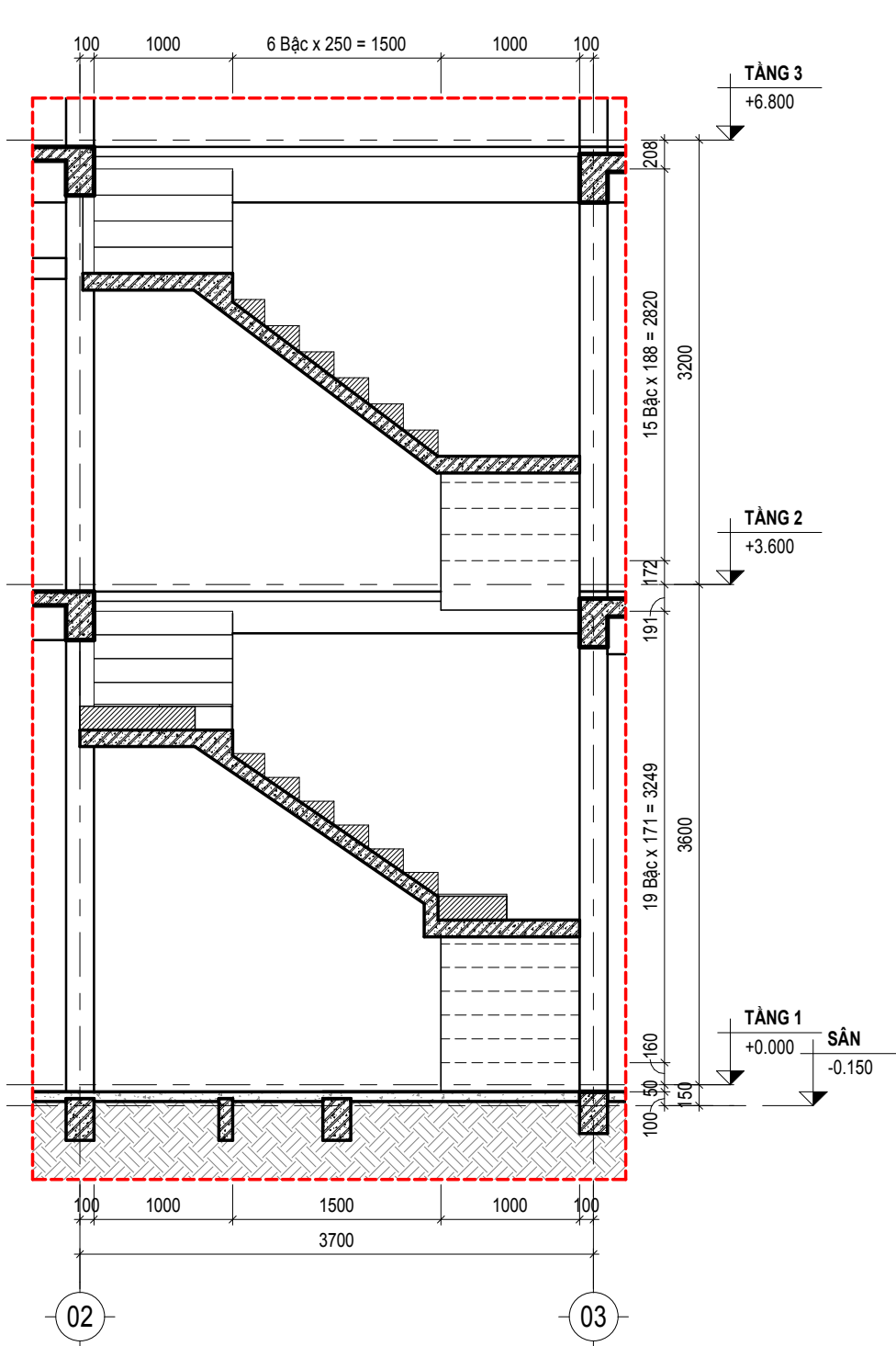
04 CHI TIẾT THANG - MẶT CẮT 04 TỶ LỆ 1 : 50
