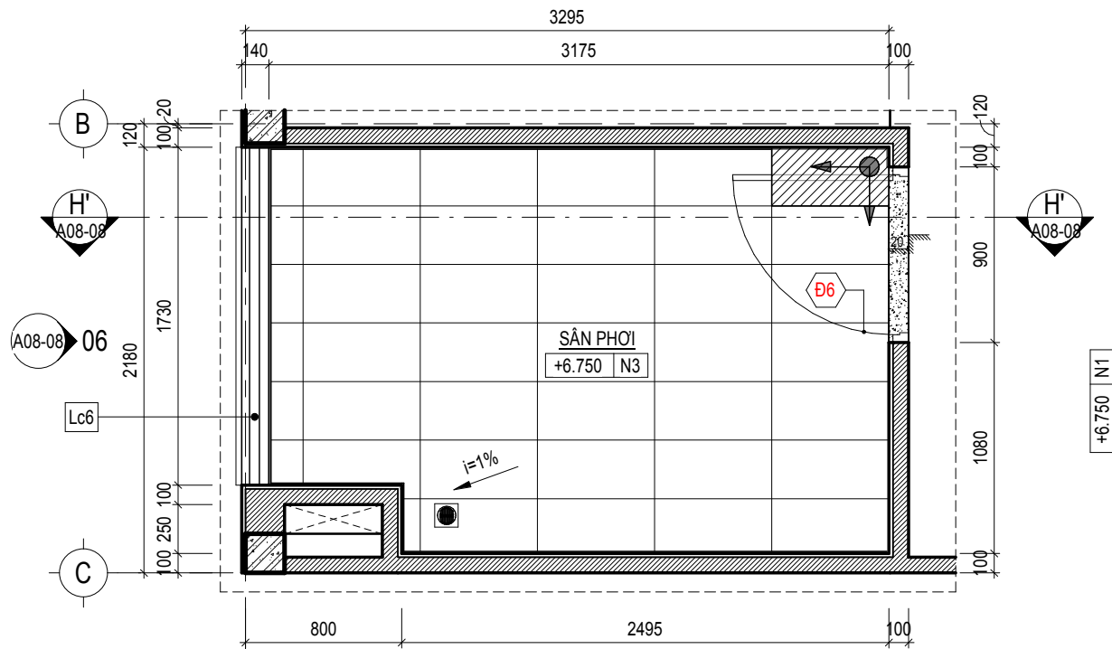
CT SÂN PHƠI TẦNG 3 - MẶT BẰNG TỶ LỆ 1 : 35
