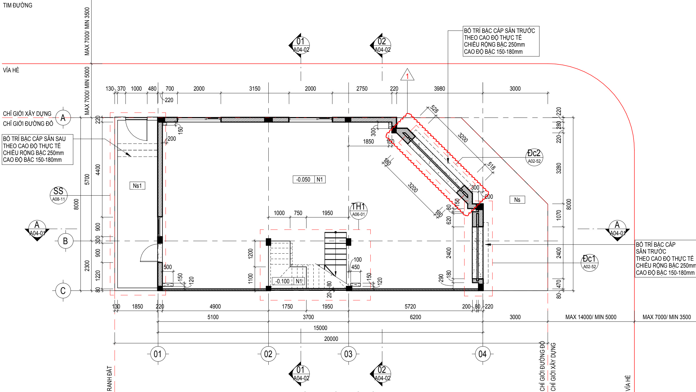
MẶT BẰNG XÂY TÔ TẦNG 1 TỶ LỆ 1 : 100
