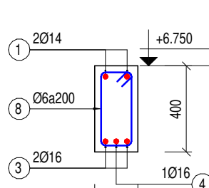
MC 5-5 3Y4 (TL: 1/25)
