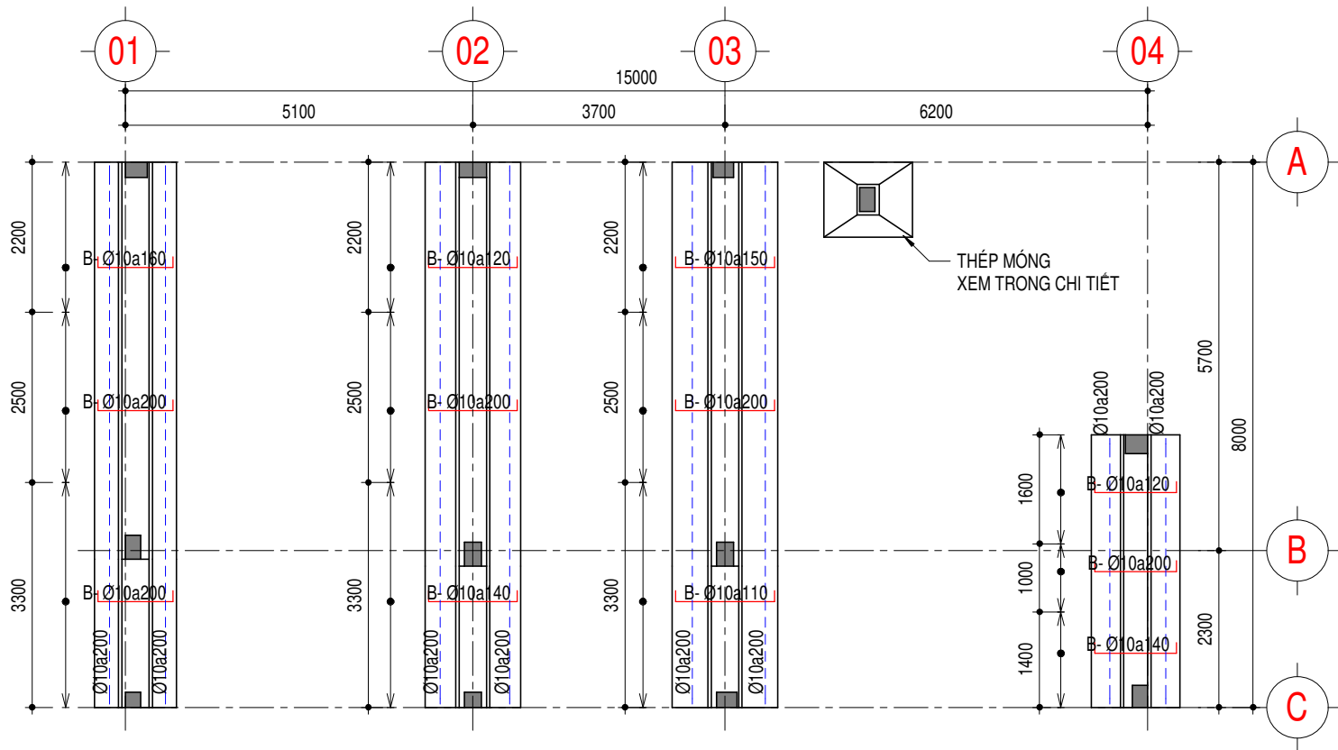
MẶT BẰNG BỐ TRÍ THÉP ĐÁY MÓNG
