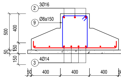
MC 5-5 PA1 - M2 (TL: 1/25)
