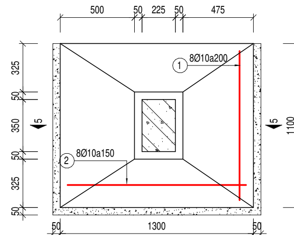
MÓNG M5 (SL=1)
