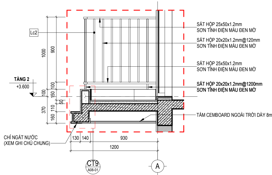
LAN CAN Lc2 (ĐIỂN HÌNH) - MC B' TỶ LỆ 1:25
