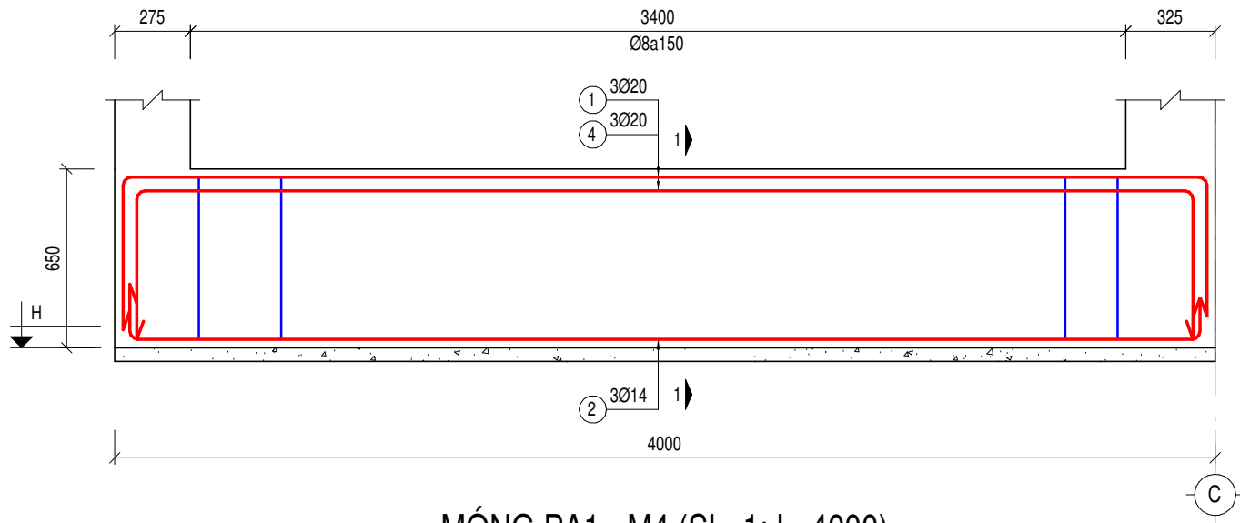
MÓNG PA1 - M4 (SL=1; L=4000)
