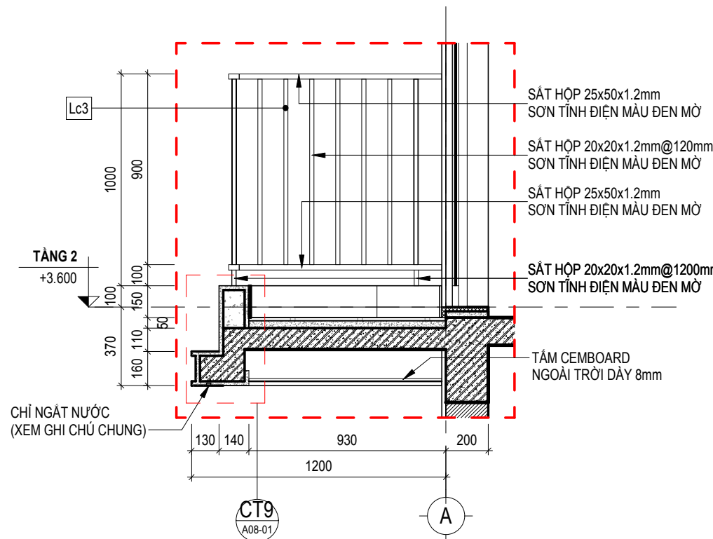
C' LAN CAN Lc3 (ĐIỂN HÌNH) - MC C' TỶ LỆ 1 : 25
