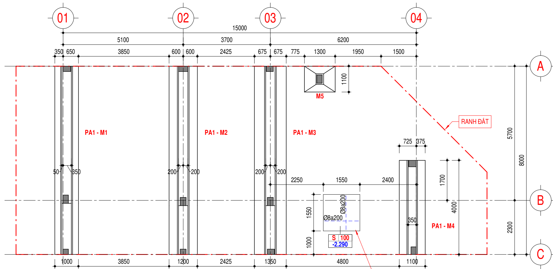
MẶT BẰNG BỐ TRÍ MÓNG
