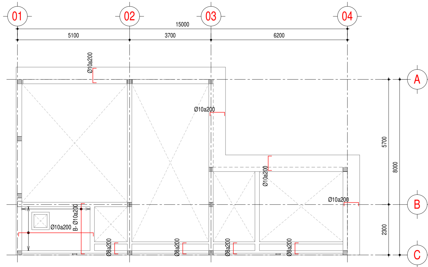
MẶT BẰNG THÉP SÀN MÁI - LỚP TRÊN
