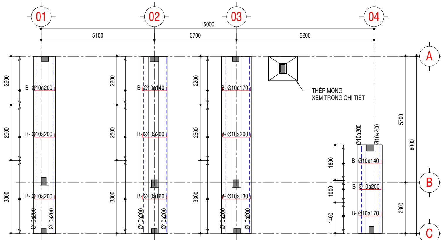
MẶT BẰNG BỐ TRÍ THÉP ĐÁY MÓNG
