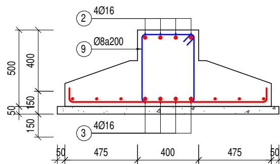
MC 5-5 PA1 - M3 (TL: 1/25)
