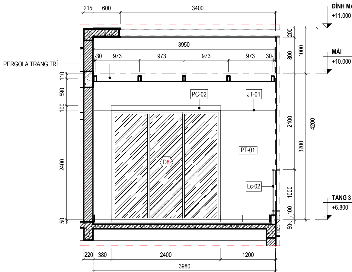
CHI TIẾT LAM MÁI - MẶT CẮT G' - 03 TỶ LỆ 1:50
