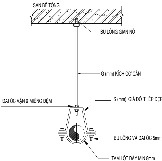
CHI TIẾT TREGO ØNG
