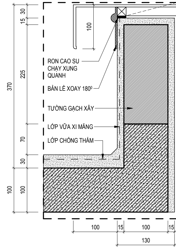
CT13 - LIÊN KẾT BẢN LỀ NẮP THẢM MÁI
