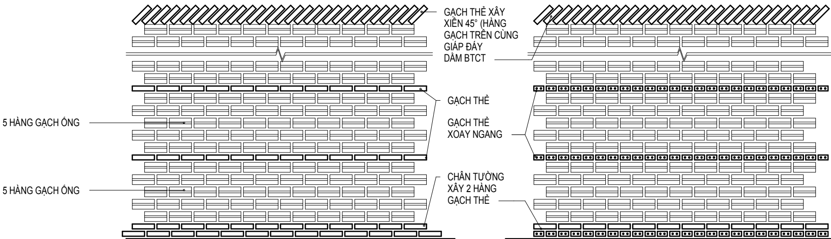
CHI TIẾT ĐIỂN HÌNH XÂY TƯỜNG 100mm
