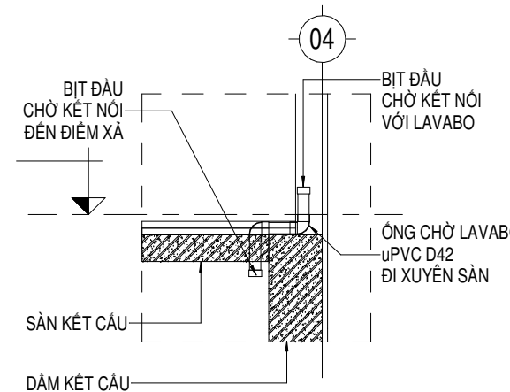
MẶT CẮT A-A TỶ LỆ 1 : 25
