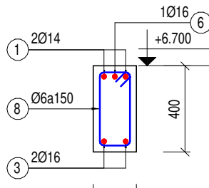
MC 2-2 3Y4 (TL: 1/25)
