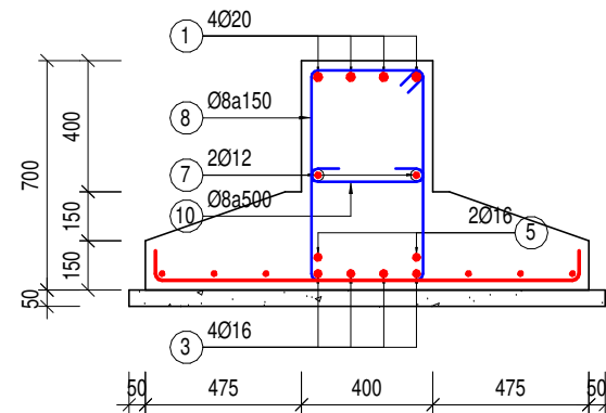
MC 3-3 PA1 - M3 (TL: 1/25)
