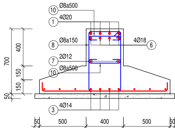
MC 2-2 PA2 - M2 (TL: 1/25)
