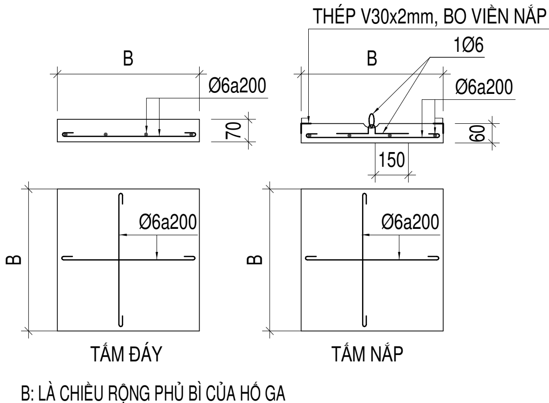
CHI TIẾT HỒ GA, TỶ LỆ 1/25
