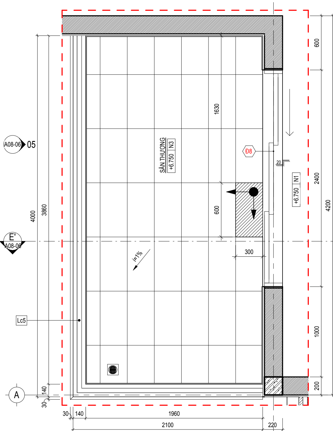
ST A02-53 CT SÂN THƯƠNG TẦNG 3 - MẶT BẰNG TỶ LỆ 1 : 25
