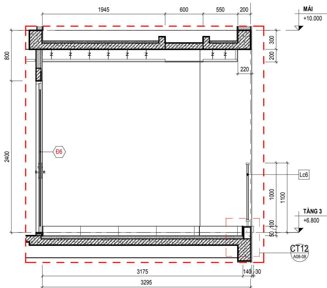
CT SÂN PHƠI TẦNG 3 - MẶT CẮT H' TỶ LỆ 1 : 35
