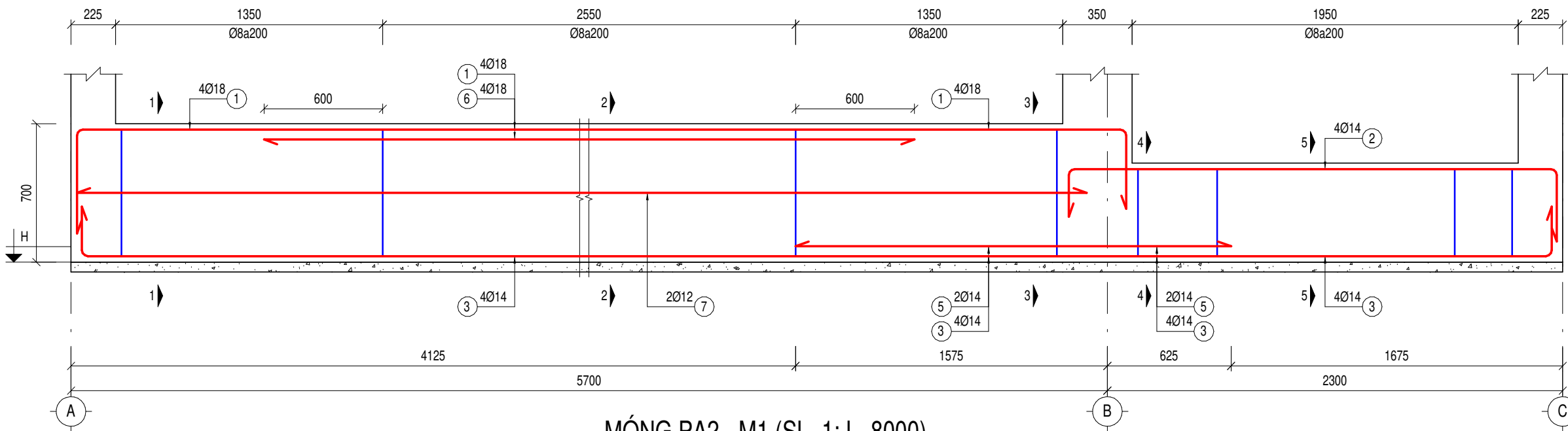
MÓNG PA2 - M1 (SL=1; L=8000)
