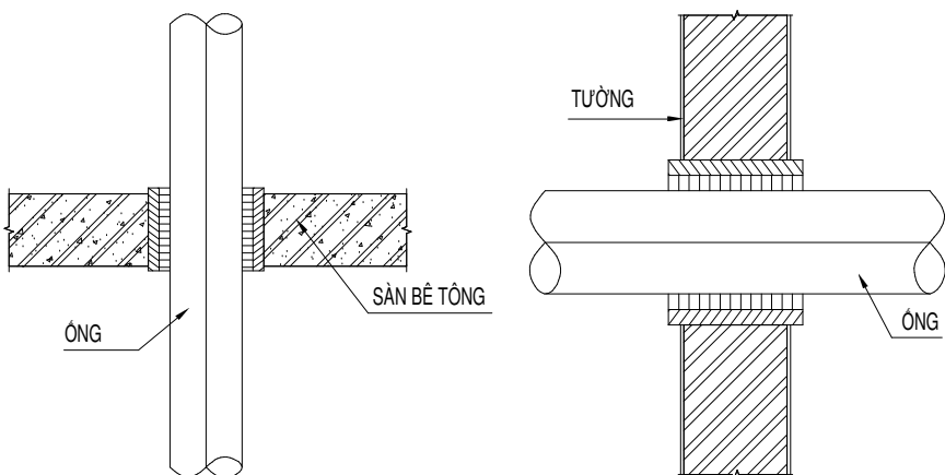
CHI TIẾT ØNG XUYỀN SÀN, TƯỜNG ĐIỂN HÌNH
