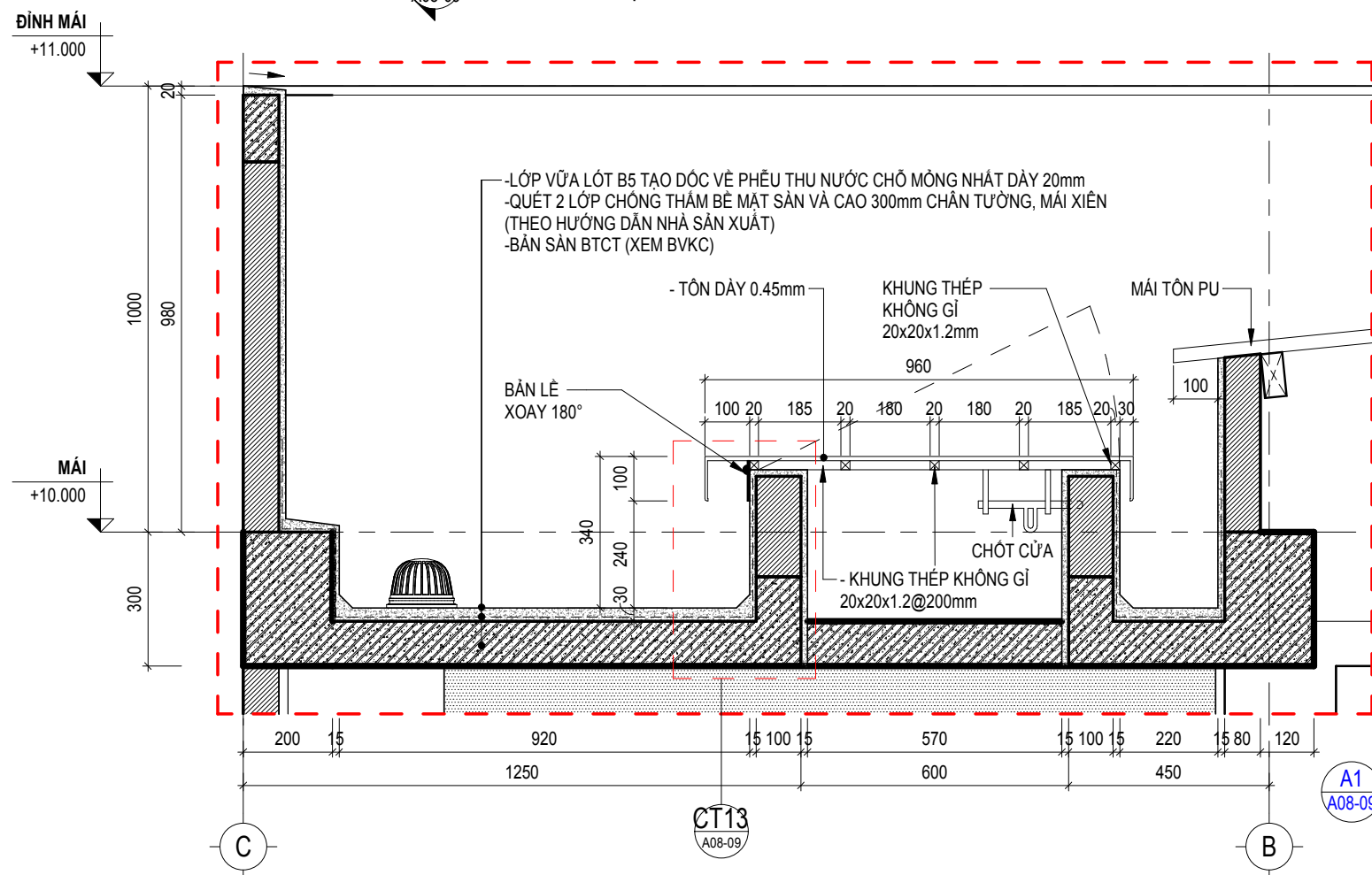
CHI TIẾT NẮP THẢM MÁI - MẶT CẮT A1
