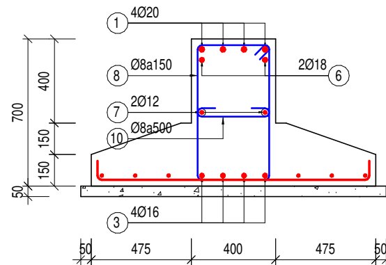
MC 2-2 PA1 - M3 (TL: 1/25)
