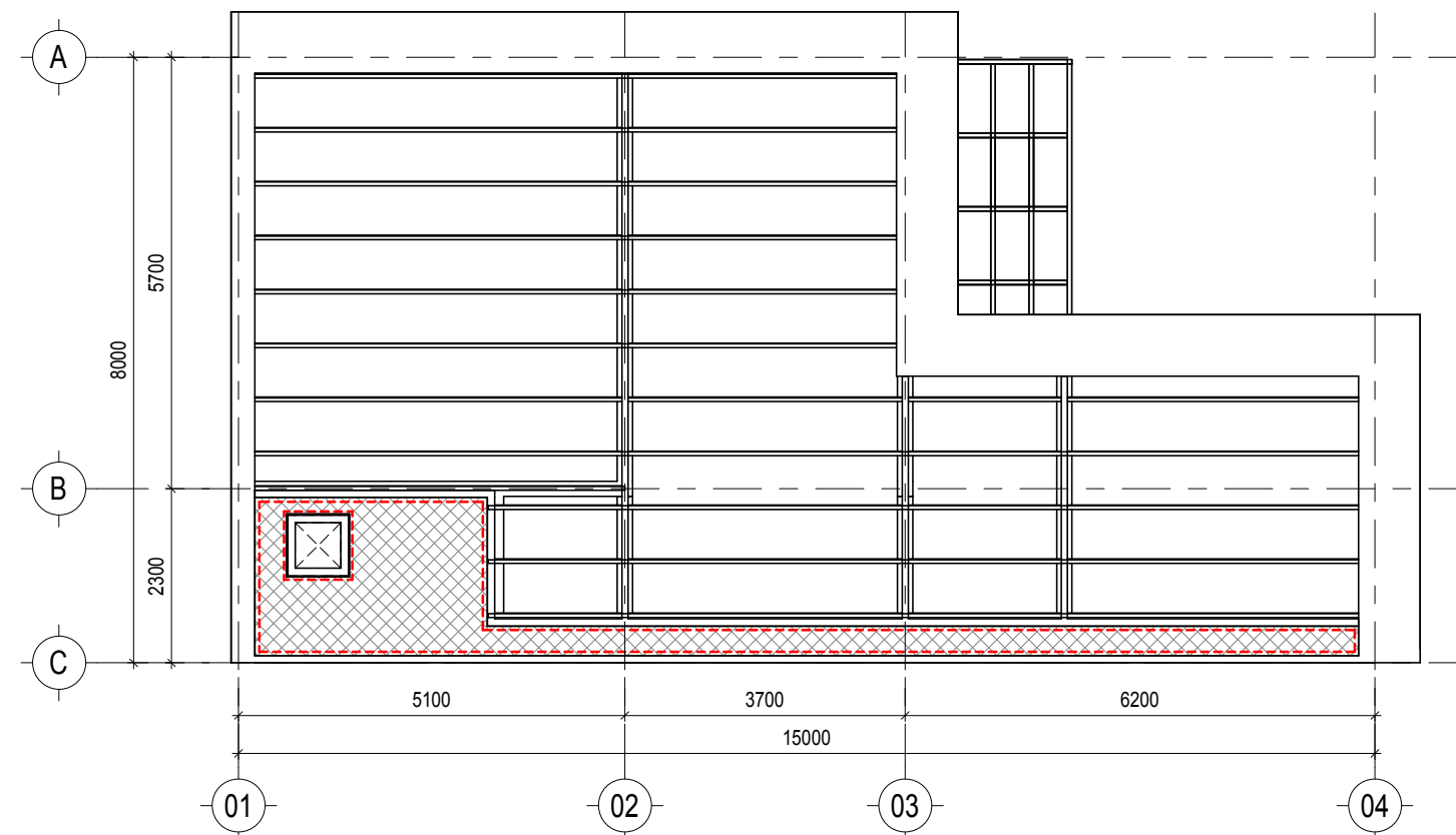
MẶT BẰNG CHỐNG THẨM MÁI
