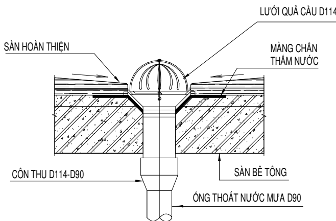
CHI TIẾT LẮP ĐẶT PHỄU THU SÀN (TREGO TRẦN)
