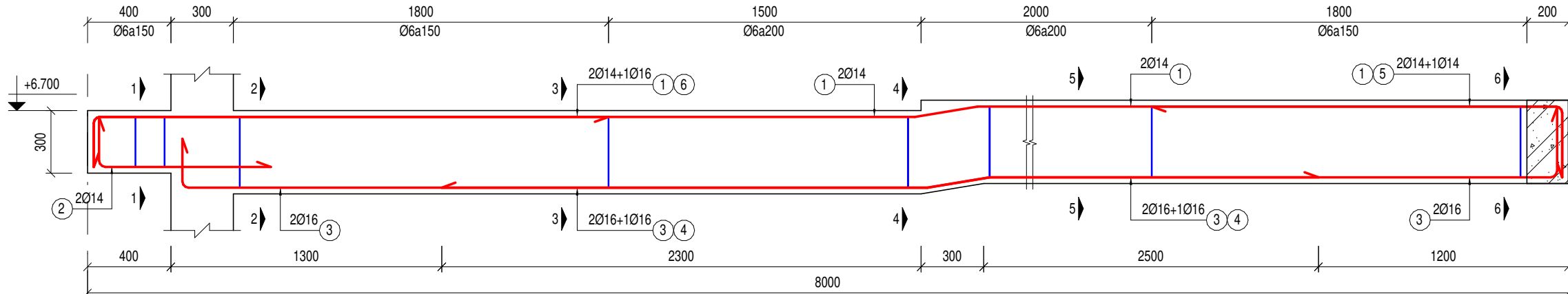
DÀM 3Y4 (SL=1; L=8000)
