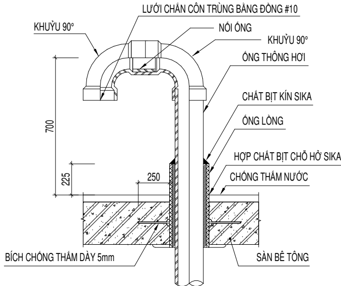
CHI TIẾT ØNG THÔNG HƠI VƯỢT MÁI
