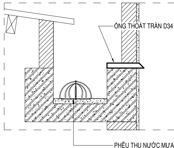
CHI TIẾT ØNG THOÁT TRẦN SÊ NÔ
