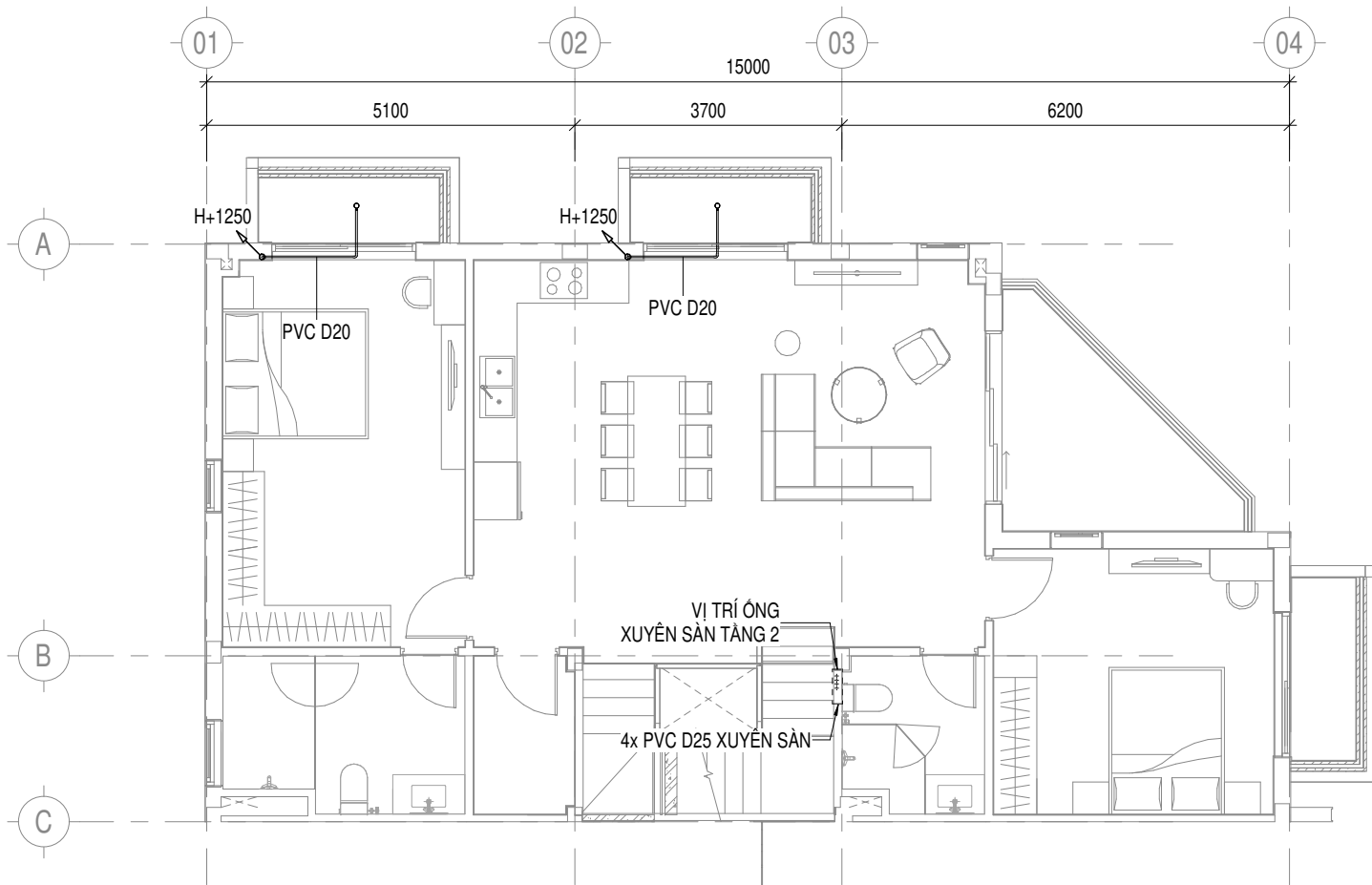
MẶT BẰNG CẤP NGUỒN, THÔNG TIN LIÊN LẠC TẦNG 2 TỶ LỆ 1 : 100
