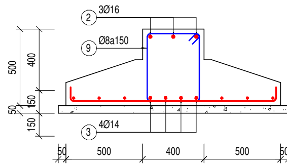
MC 5-5 PA2 - M2 (TL: 1/25)
