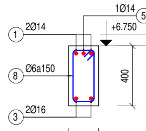
MC 6-6 3Y4 (TL: 1/25)
