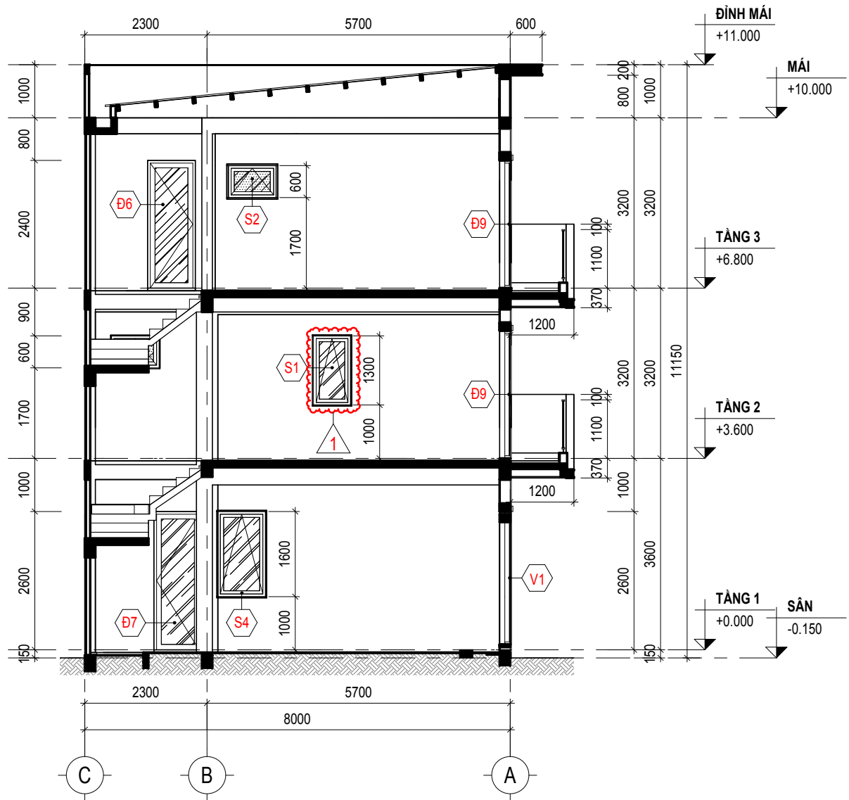
MẶT CẮT 1-1 TỶ LỆ 1:100
