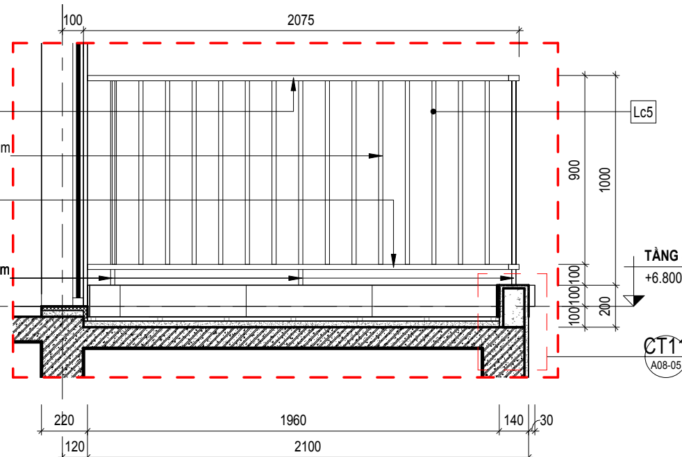
E' A08-06 LAN CAN Lc5 - MẶT CẮT E' TỶ LỆ 1 : 25
