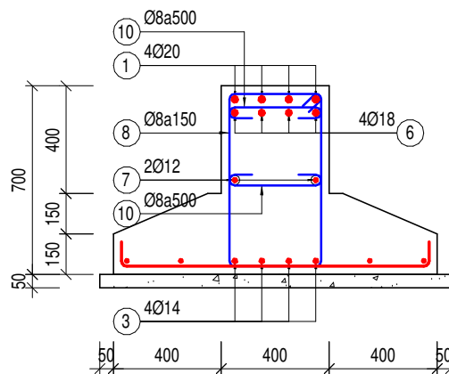
MC 2-2 PA1 - M2 (TL: 1/25)
