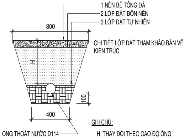
CHI TIẾT PHUI ĐÀO CHO ØNG THOÁT NƯỚC
