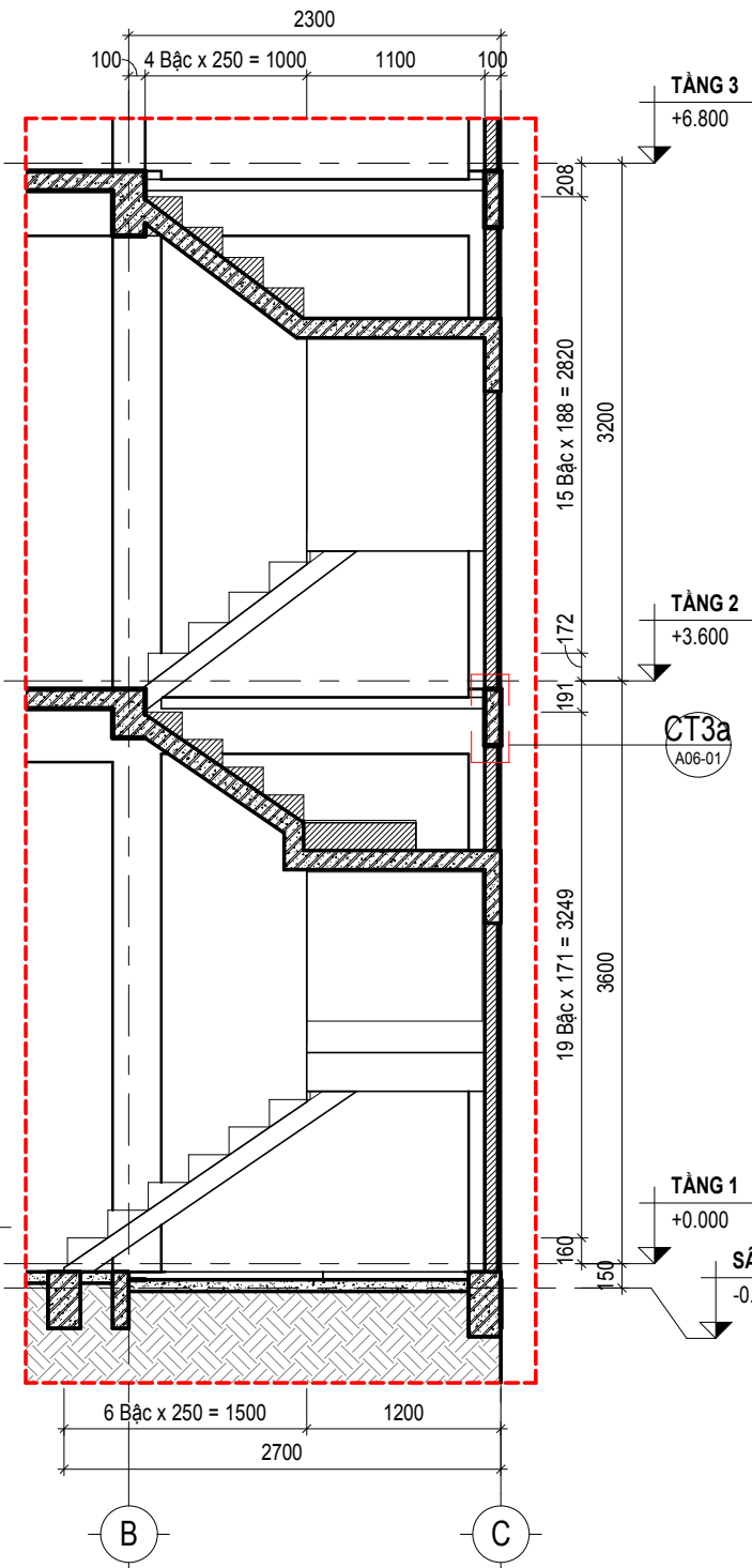
05 CHI TIẾT THANG - MẶT CẮT 5 TỶ LỆ 1 : 50
