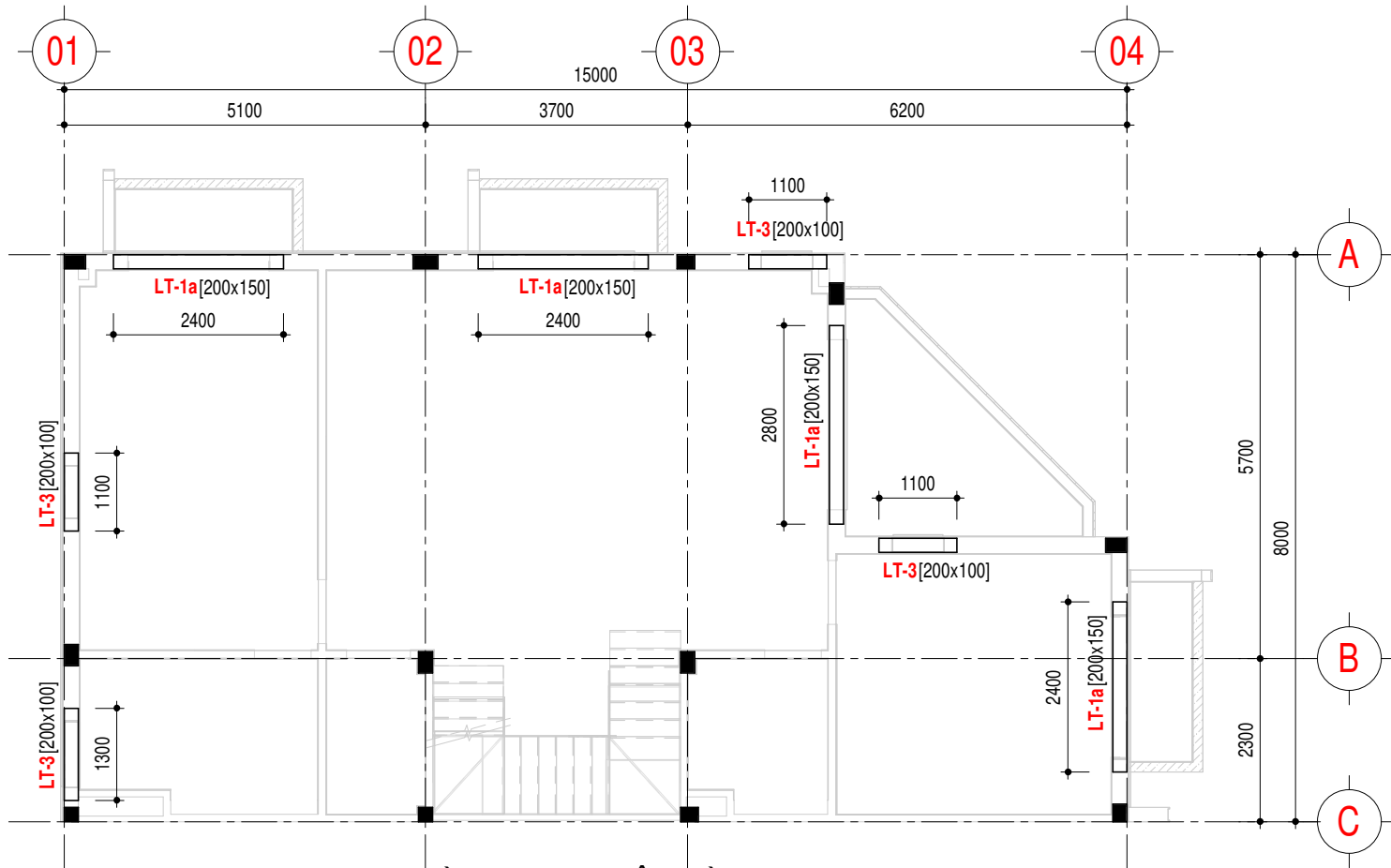
MẶT BẰNG LANH TÔ - TẦNG 2
