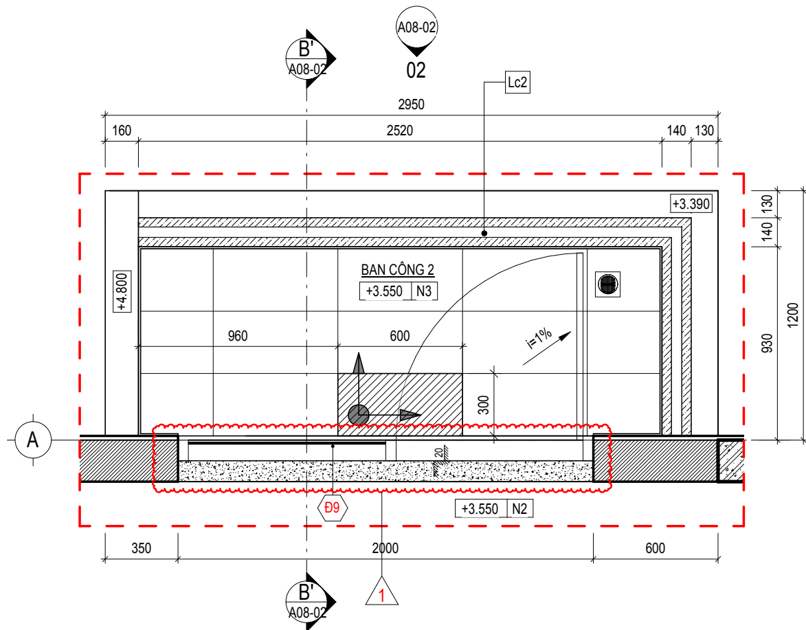
CT BAN CÔNG 2 (ĐIỂN HÌNH) - MẶT BẰNG TỶ LỆ 1:25
