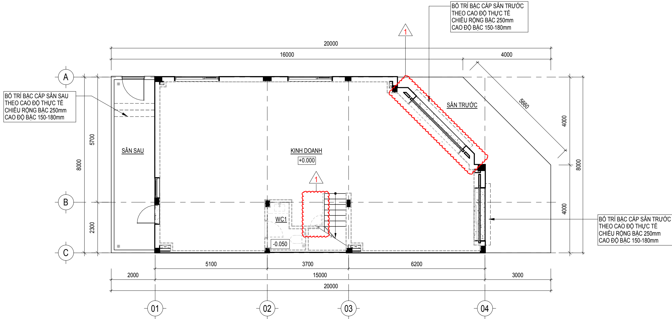
MB ĐỊNH HƯỚNG CÔNG NĂNG TẦNG 1 TỶ LỆ 1 : 100
