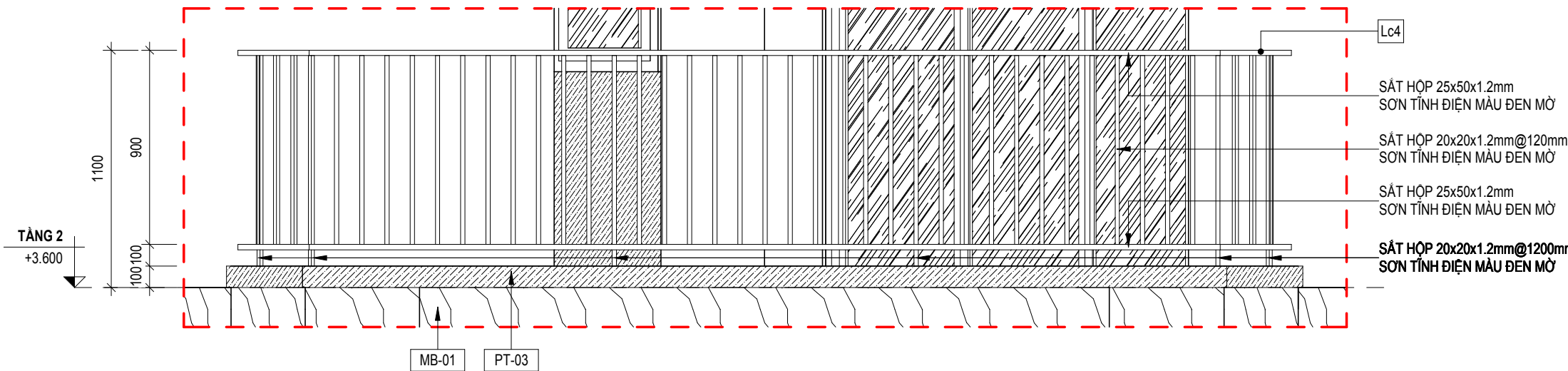
04 LAN CAN Lc4 - MĐ 04 A08-04 TỶ LỆ 1:25
