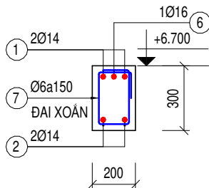
MC 1-1 3Y4 (TL: 1/25)
