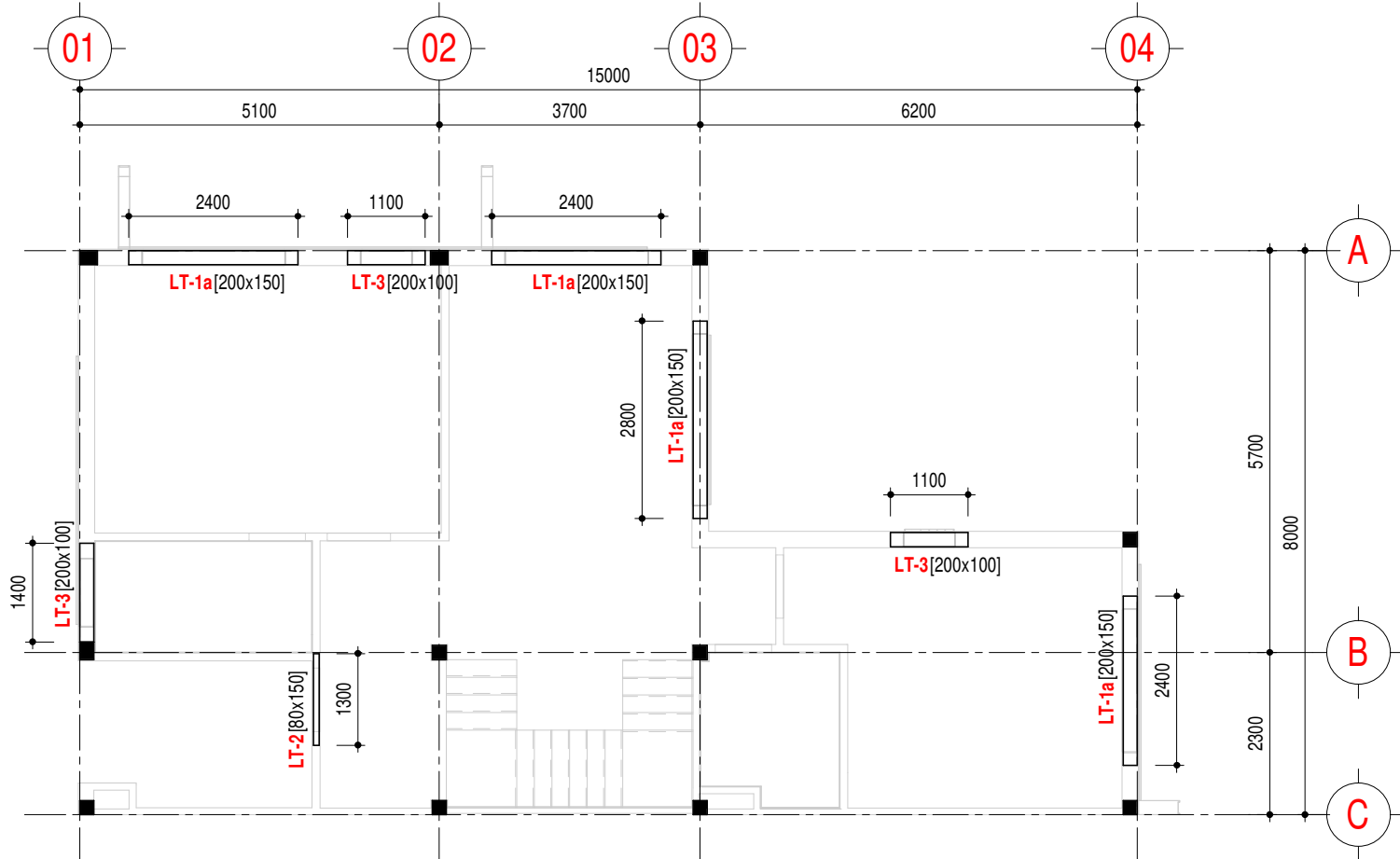
MẶT BẰNG LANH TÔ - TẦNG 3
