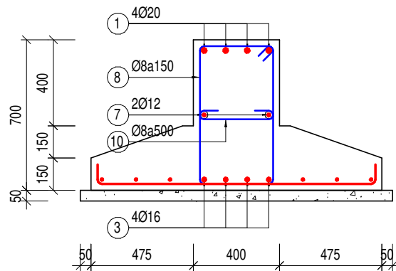
MC 1-1 PA1 - M3 (TL: 1/25)
