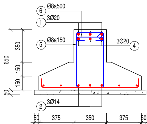
MÓNG PA1 - M4 (SL=1; L=4000)
