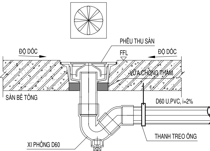
CHI TIẾT LẮP ĐẶT PHỄU THU SÀN (TREGO TRẦN)
