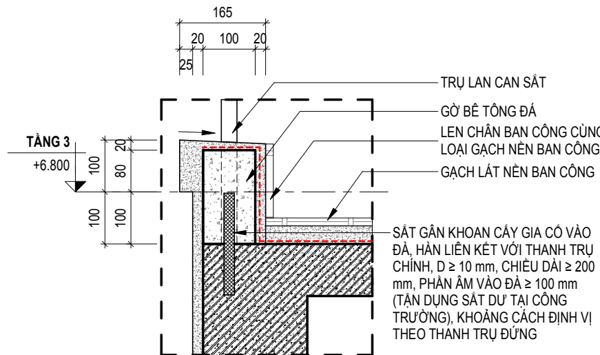
CT11 - CT GỜ CHỈ BAN CÔNG A08-04 TỶ LỆ 1:10
