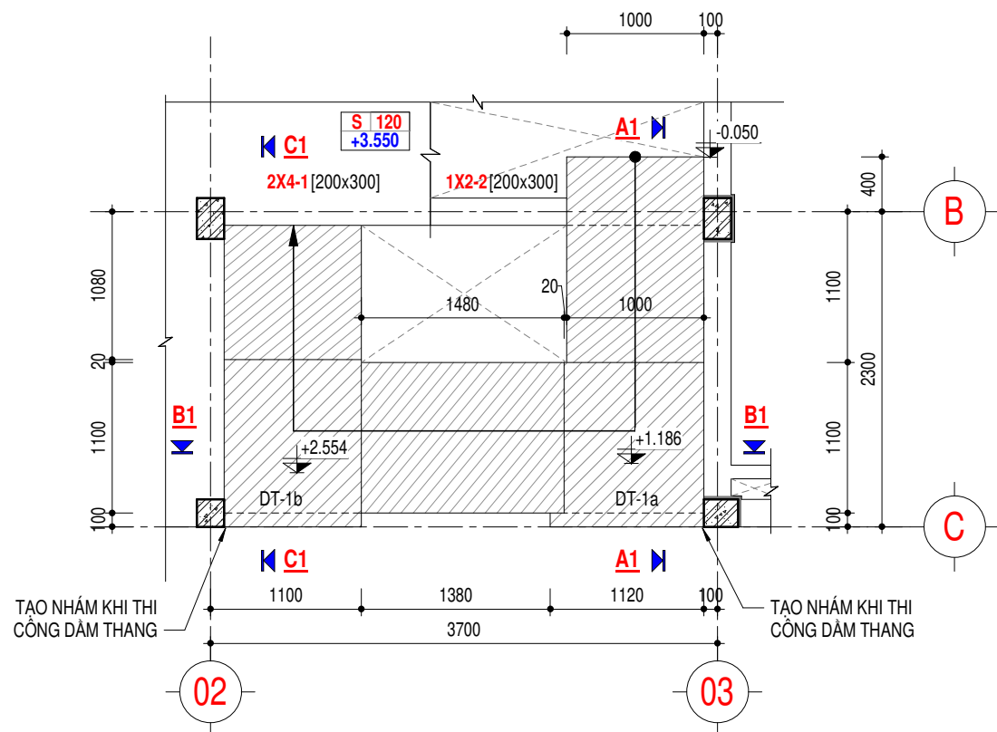
MẶT BẰNG CẦU THANG TẦNG 1 - TẦNG 2
