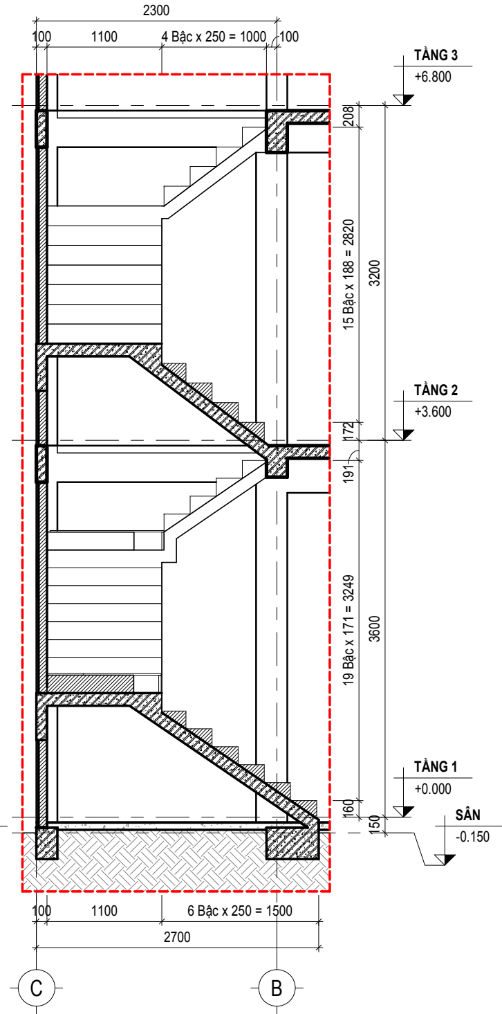
06 CHI TIẾT THANG - MẶT CẮT 6 TỶ LỆ 1 : 50
