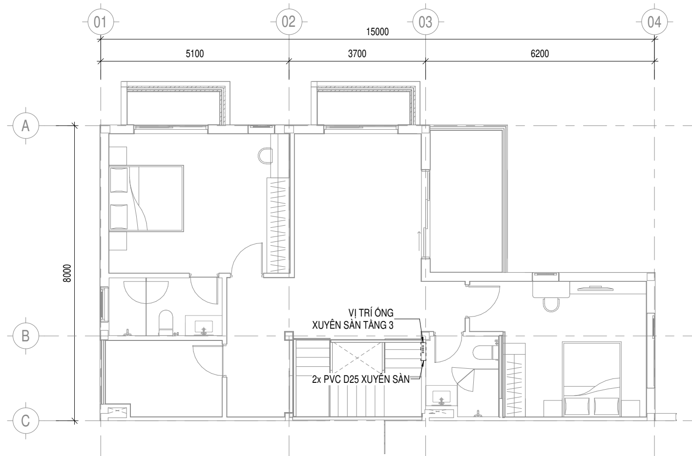
MẶT BẰNG CẤP NGUỒN, THÔNG TIN LIÊN LẠC TẦNG 3 TỶ LỆ 1 : 100
