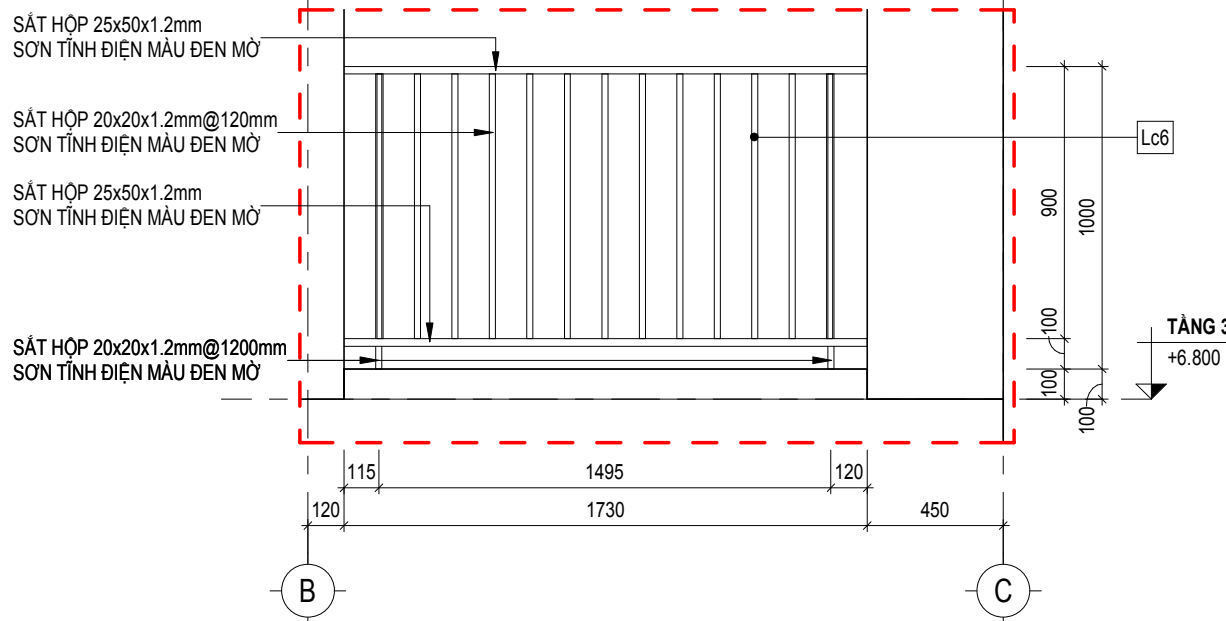
LAN CAN Lc6 - MẶT ĐỨNG 06 TỶ LỆ 1 : 25
