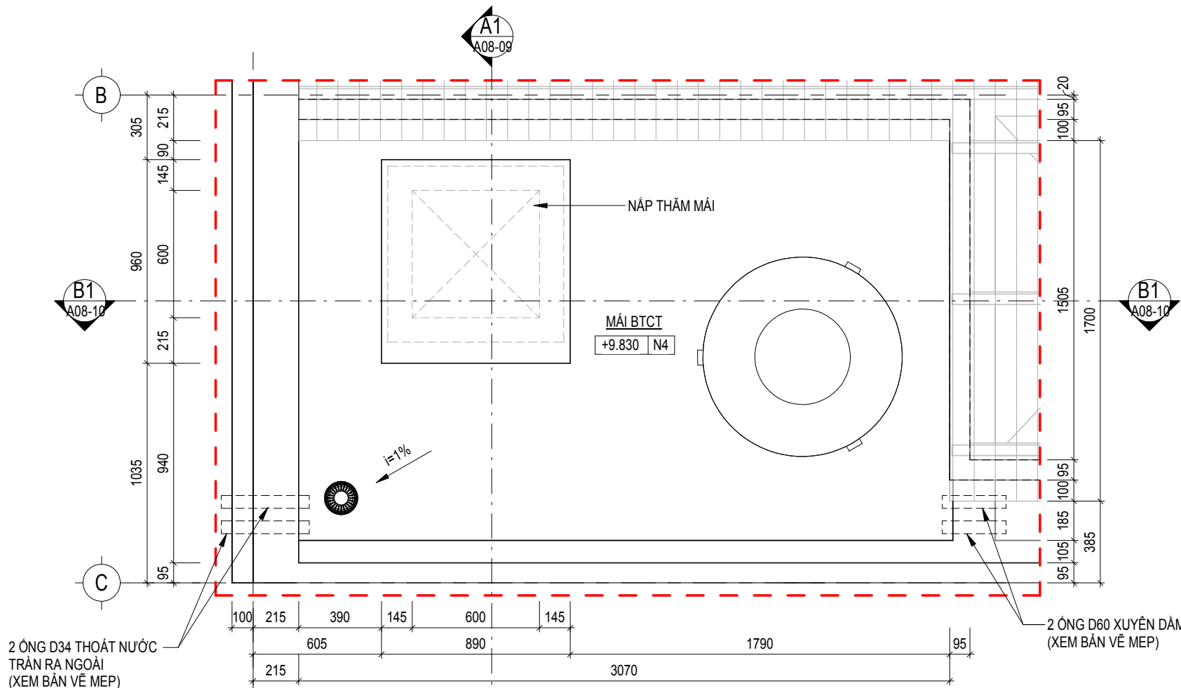
CHI TIẾT NẮP THẢM MÁI - MẶT BẰNG
