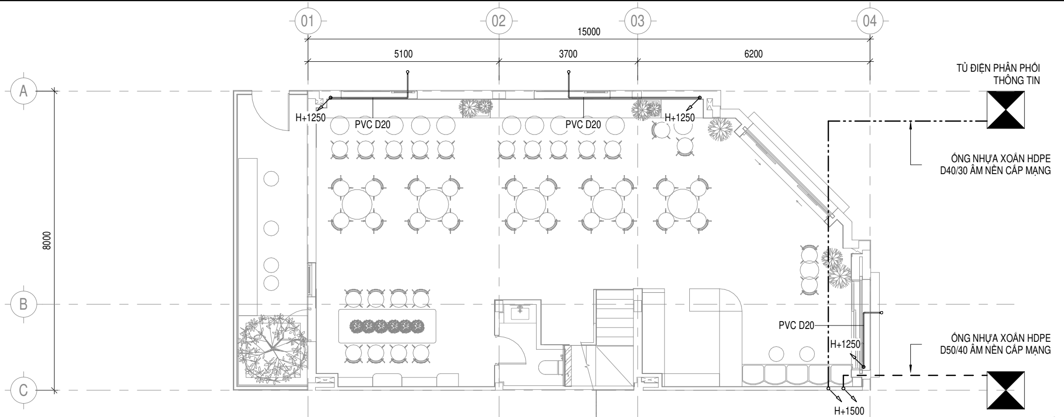
MẶT BẰNG CẤP NGUỒN, THÔNG TIN LIÊN LẠC TẦNG 1 TỶ LỆ 1 : 100
