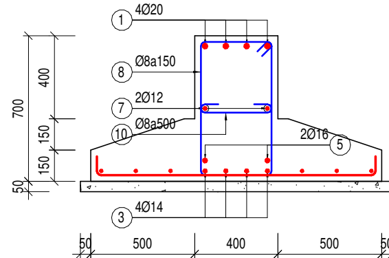
MC 3-3 PA2 - M2 (TL: 1/25)
