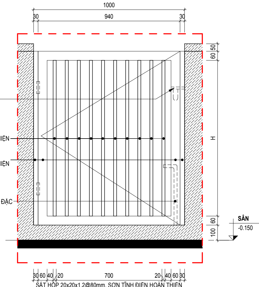
CT15 A08-12 CT15 - CHI TIẾT CỔNG RÀO TỶ LỆ 1 : 15
