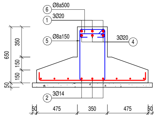
MÓNG PA2 - M4 (SL=1; L=4000)
