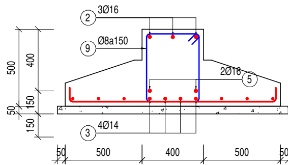
MC 4-4 PA2 - M2 (TL: 1/25)
